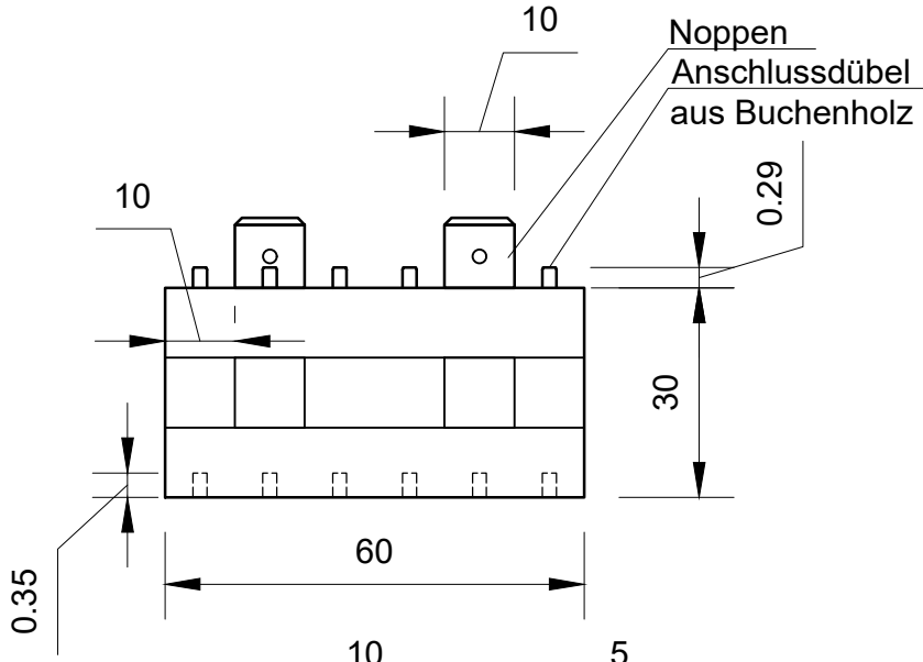
Seitenansicht
