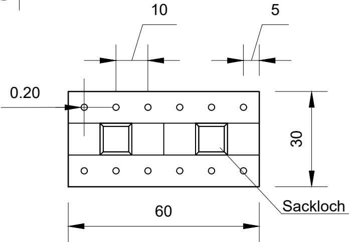
Untersicht
