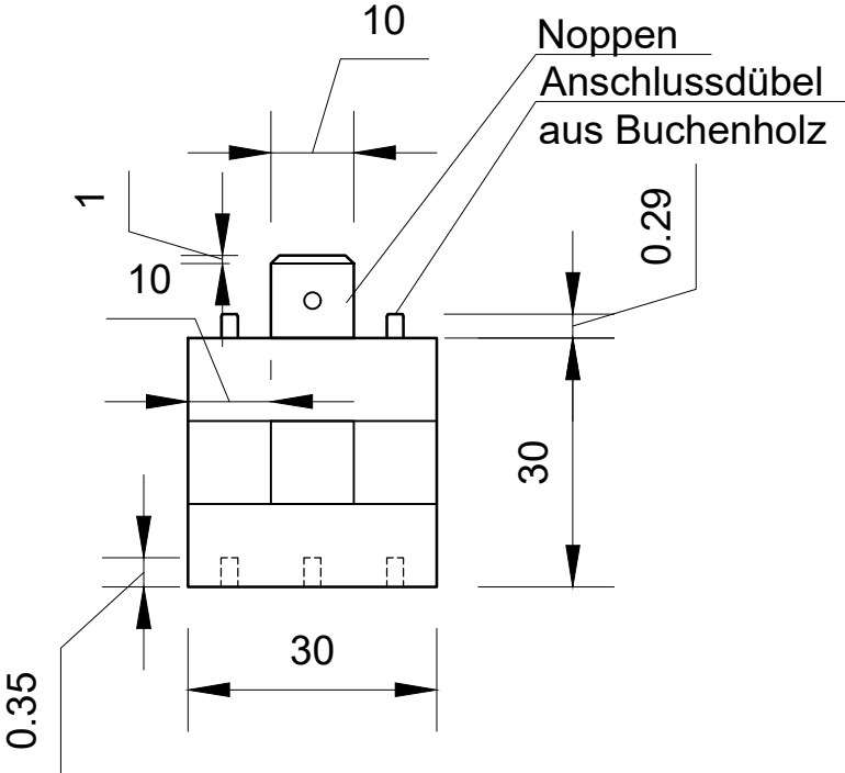
Seitenansicht
