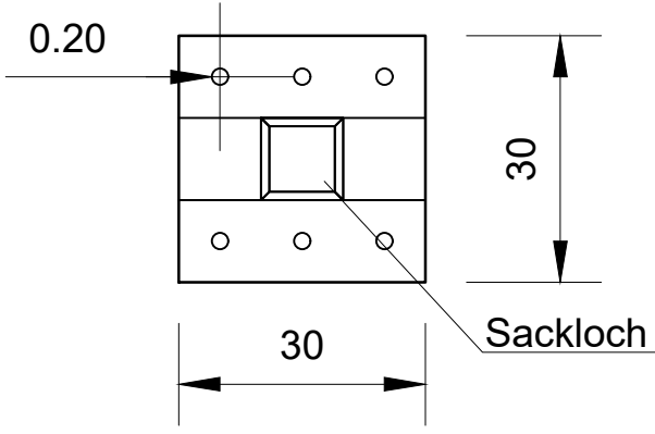
Untersicht
