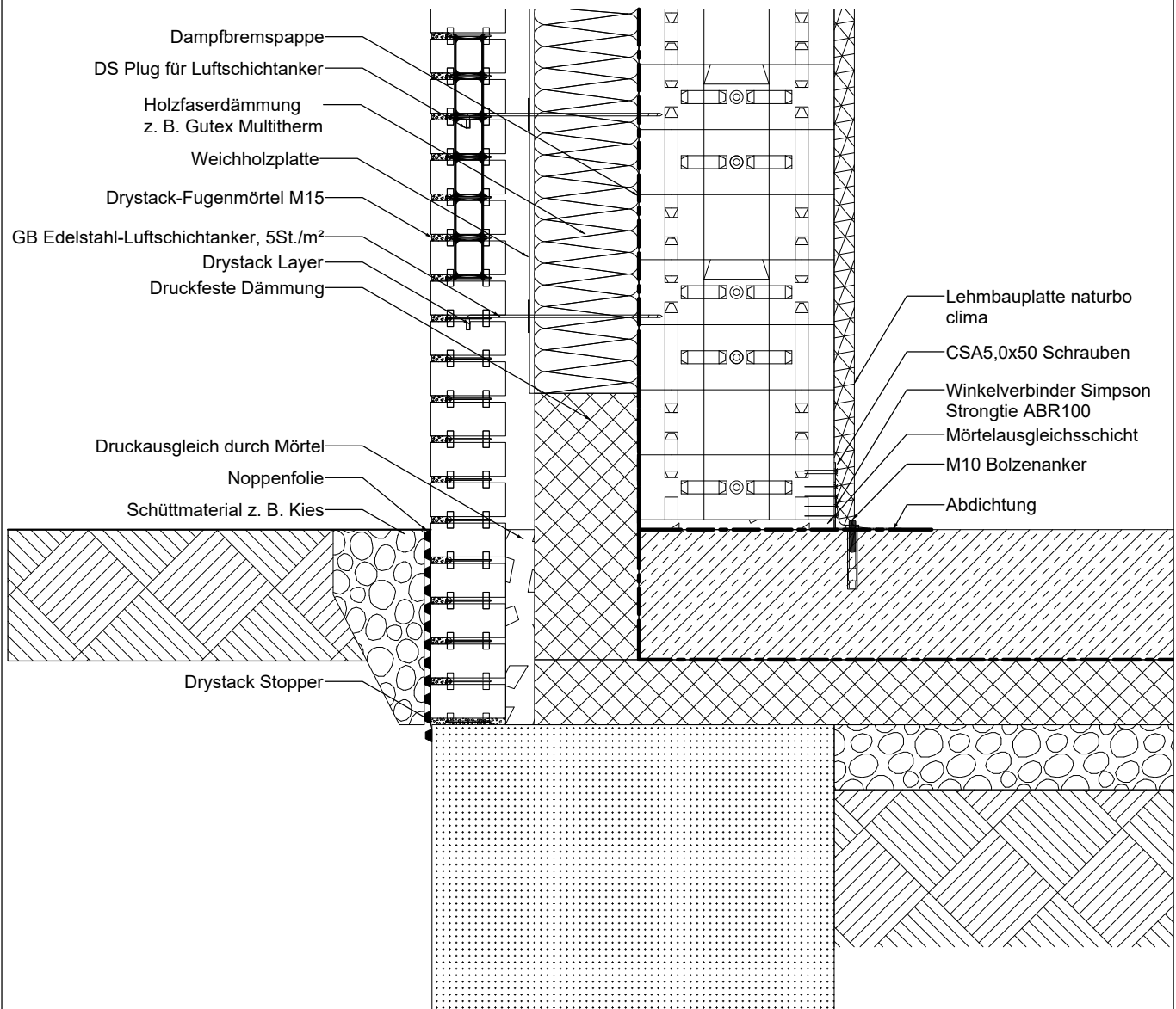
Variante 2: Detailzeichnung Sockel
